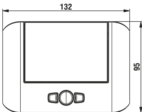
Vista frontale
